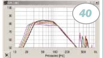
Doppelreflex-Bandpass
